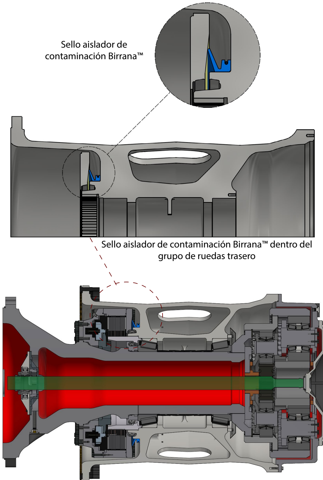
Diagrama de corte del grupo de ruedas trasero
